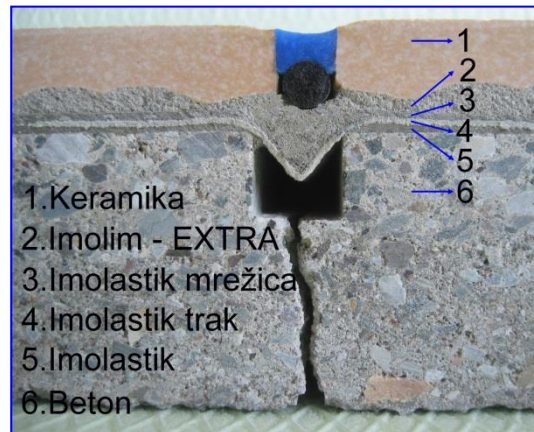
Pravilna montaža traku na dilatacijski fugi
